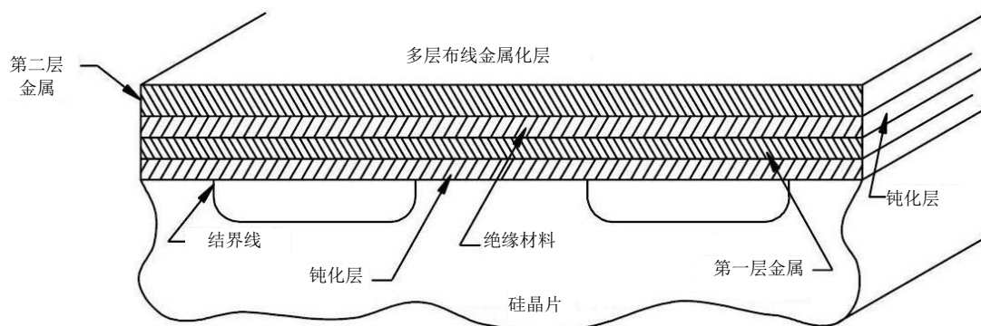
图 3 多层布线金属化层
