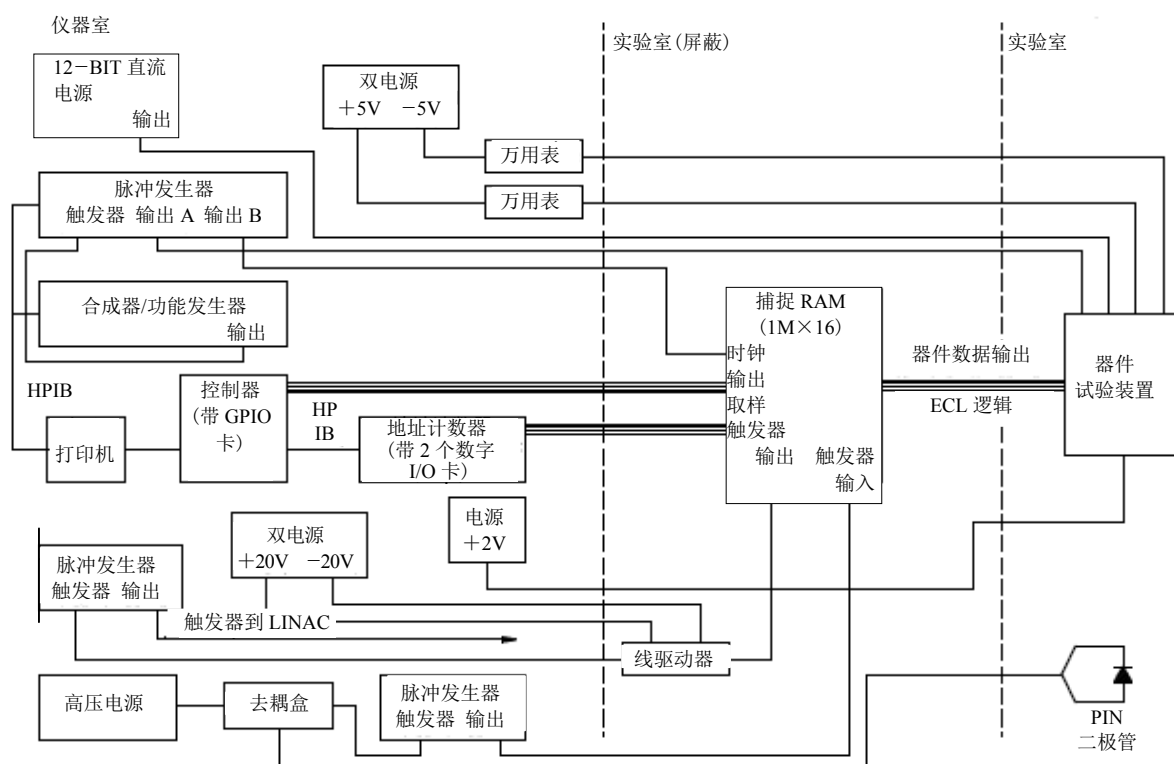
图 B.2 ADC 试验装置示例
