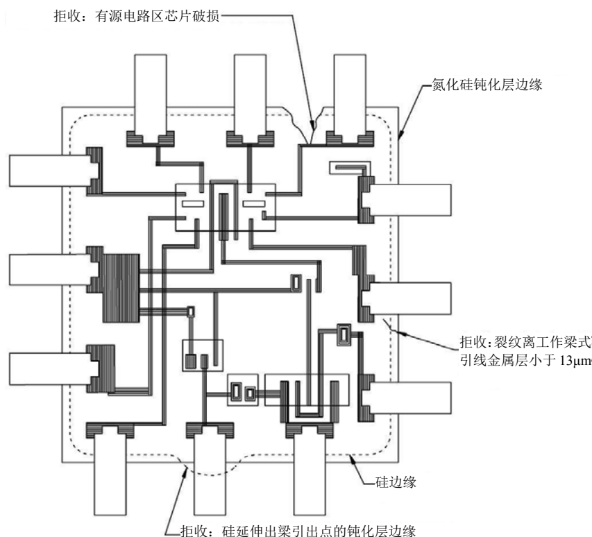
图 39 梁式引线键合芯片缺陷
