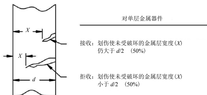
图4 S级的金属化层划伤判据
