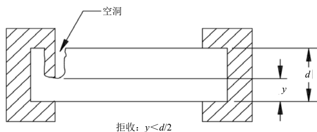
图 46 末端处空洞使电阻宽度减少的 H 级判据
