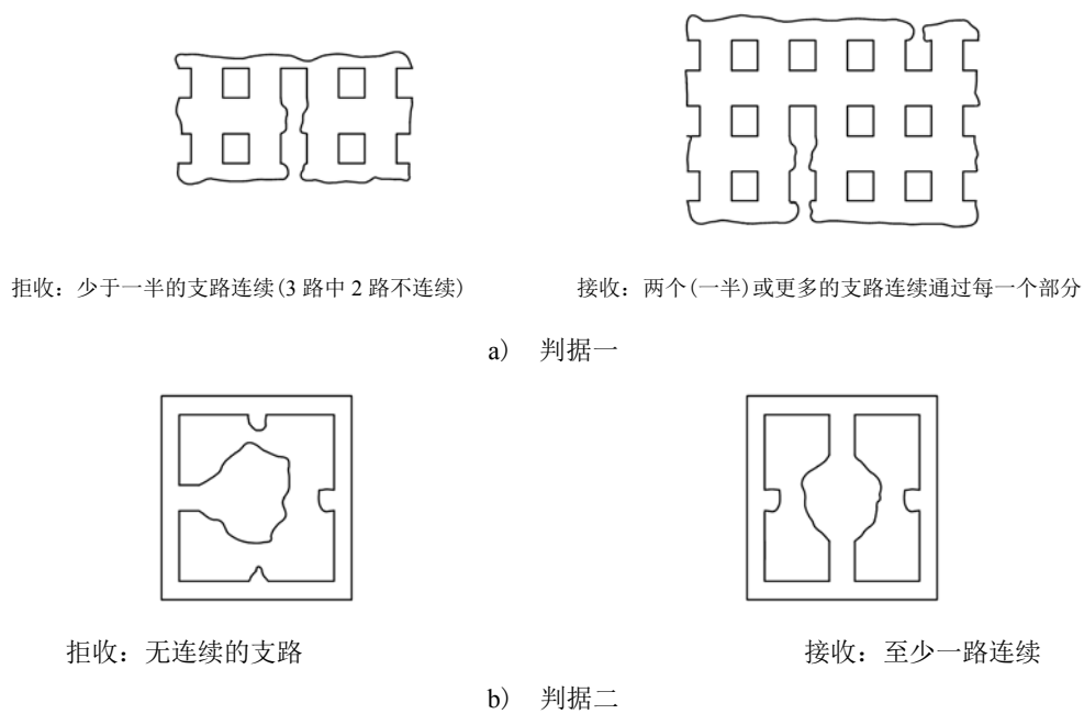
图8 网眼键合判据
