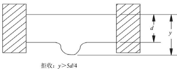
图 20 H 级电阻宽度增大判据
