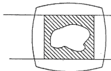
图 3 拒收的焊接区
