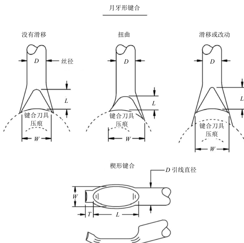
图 33 键合尺寸
