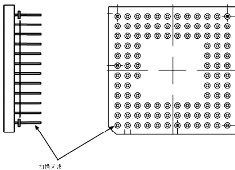
图 7 针栅阵列封装的扫描区域
