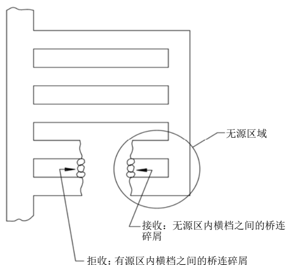
图 26 电阻阶梯结构中有源区域内横档之间的碎屑桥接判据
