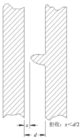
图5 H级工作金属化突出判据
