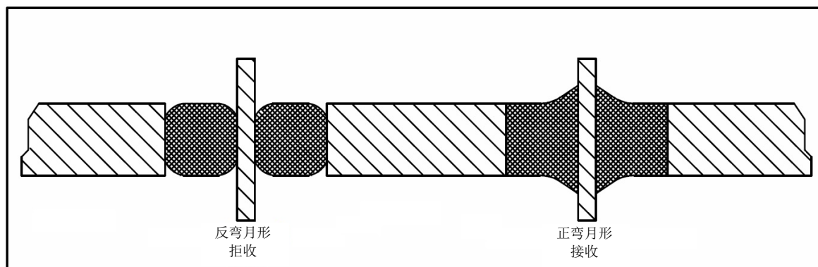
图 9 凹形密封
