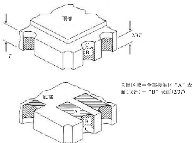
图 A.5 无引线片式载体 LCC
