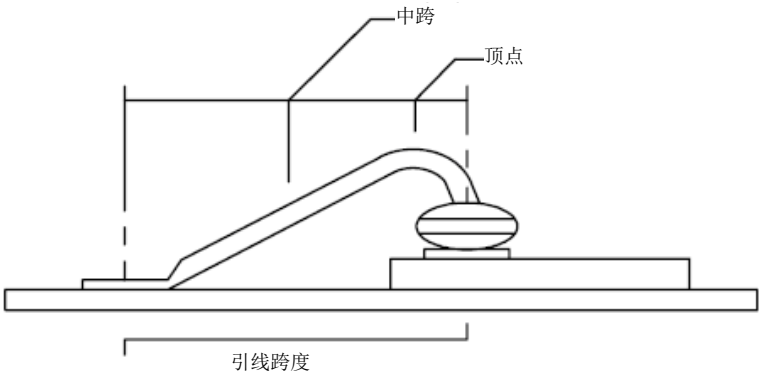
图 1 键合拉力钩子放置位置
