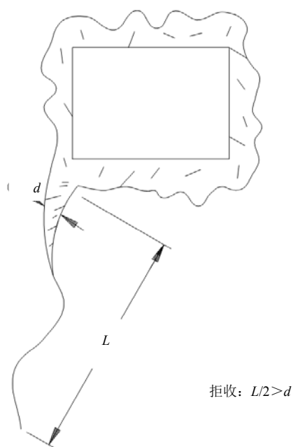
c) 粘接线判据
