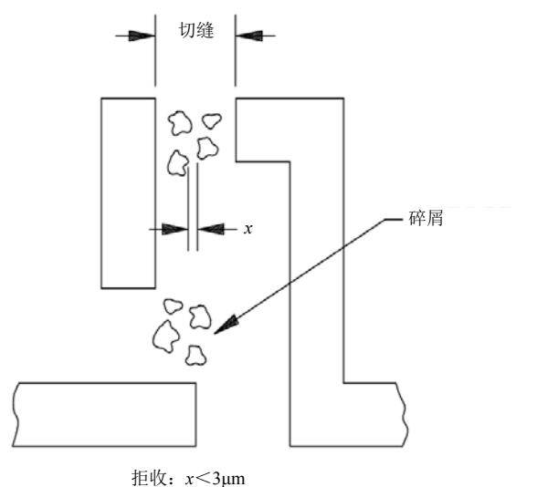
图 25 对于自钝化电阻材料电阻环状元件 H 级碎屑判据
