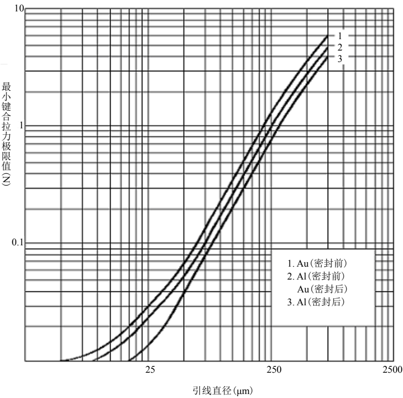
图 2 最小键合拉力极限值
