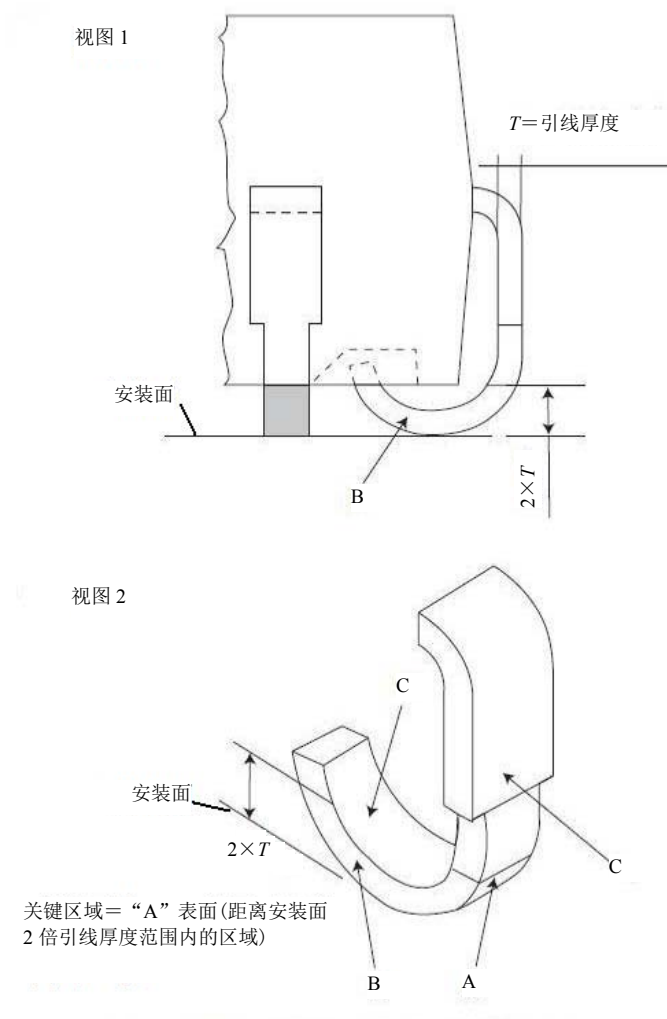
图 A.1 J形引线器件
