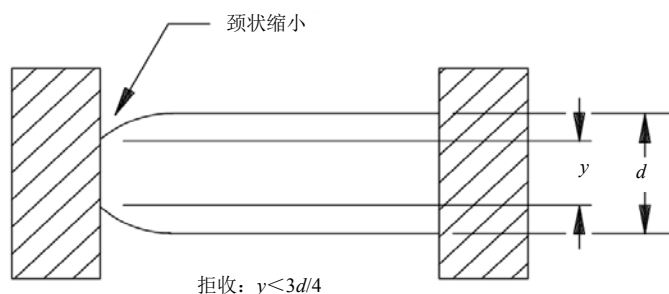
图 14 末端处径状缩小减少膜电阻宽度的 H 级判据
