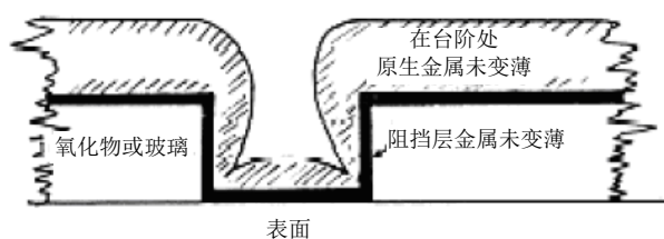
图 24 20%金属层覆盖(包括阻挡金属)
