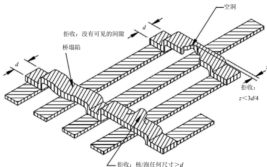
图 18 S 级和 B 级的耦合(空气)桥判据
