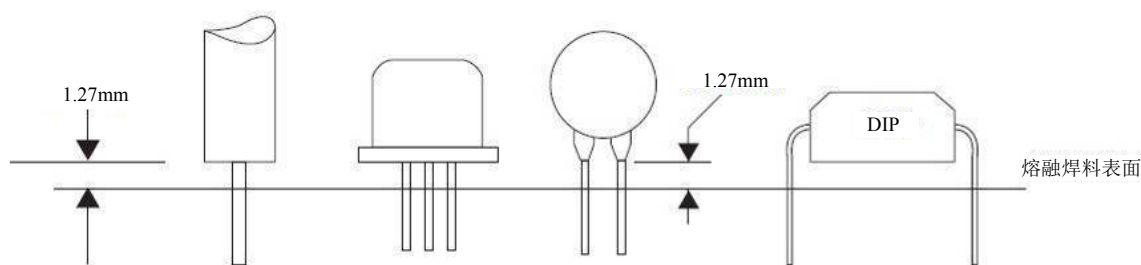
图 3 通孔安装器件的浸焊料深度
