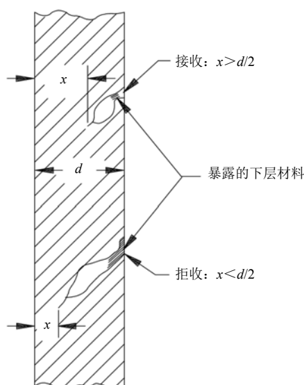
图 38 H 级金属化划伤判据
