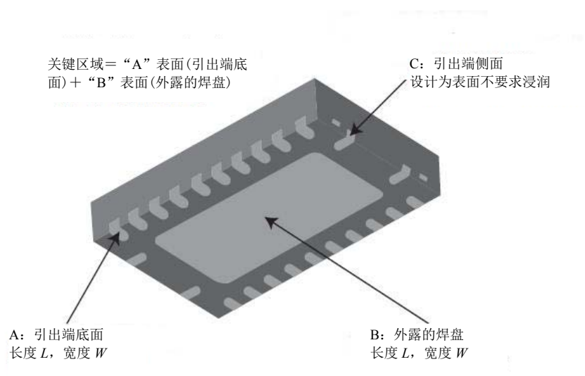
图 A.8 外露焊盘封装
