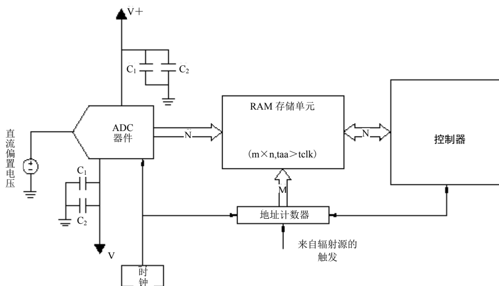
图 B.1 ADC 试验电路示例
