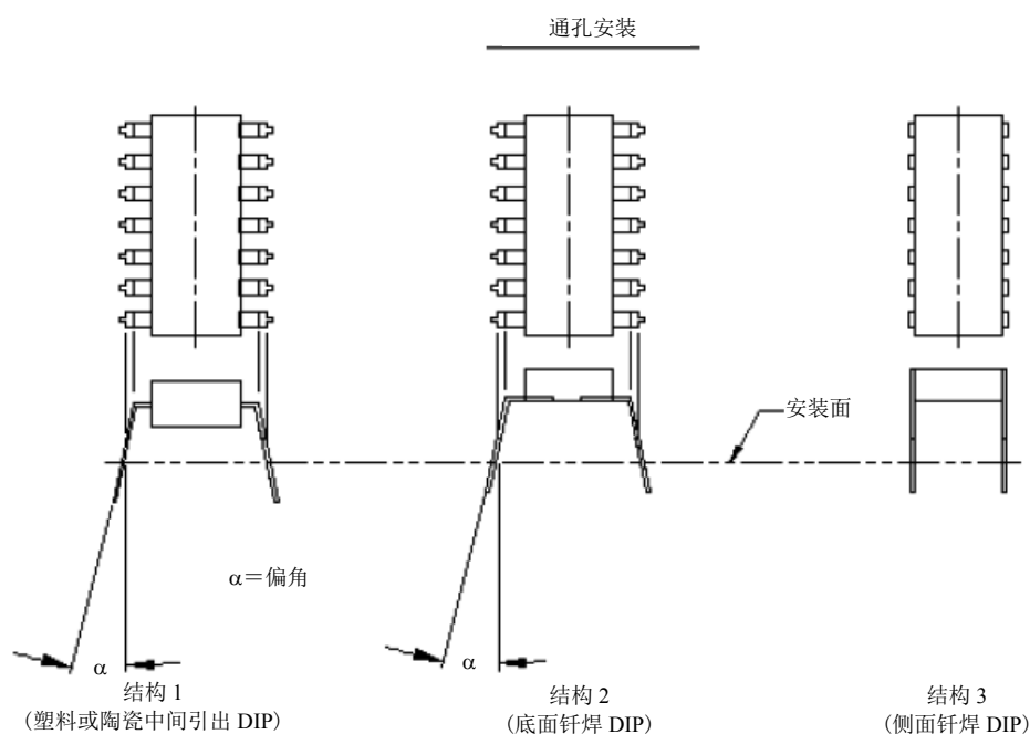
图1 封装形式
