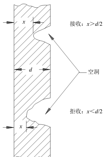
图 40 H 级金属化空洞判据
