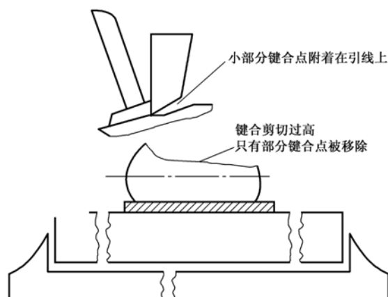
图 A. 5 跳剪
