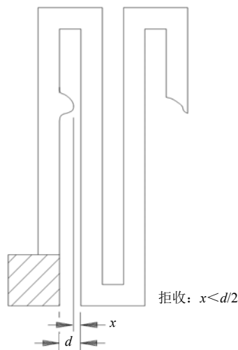
图 21 H 级电阻材料突出判据
