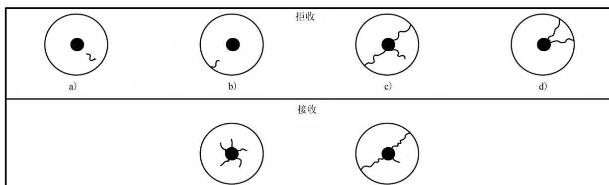
图5 径向裂纹
