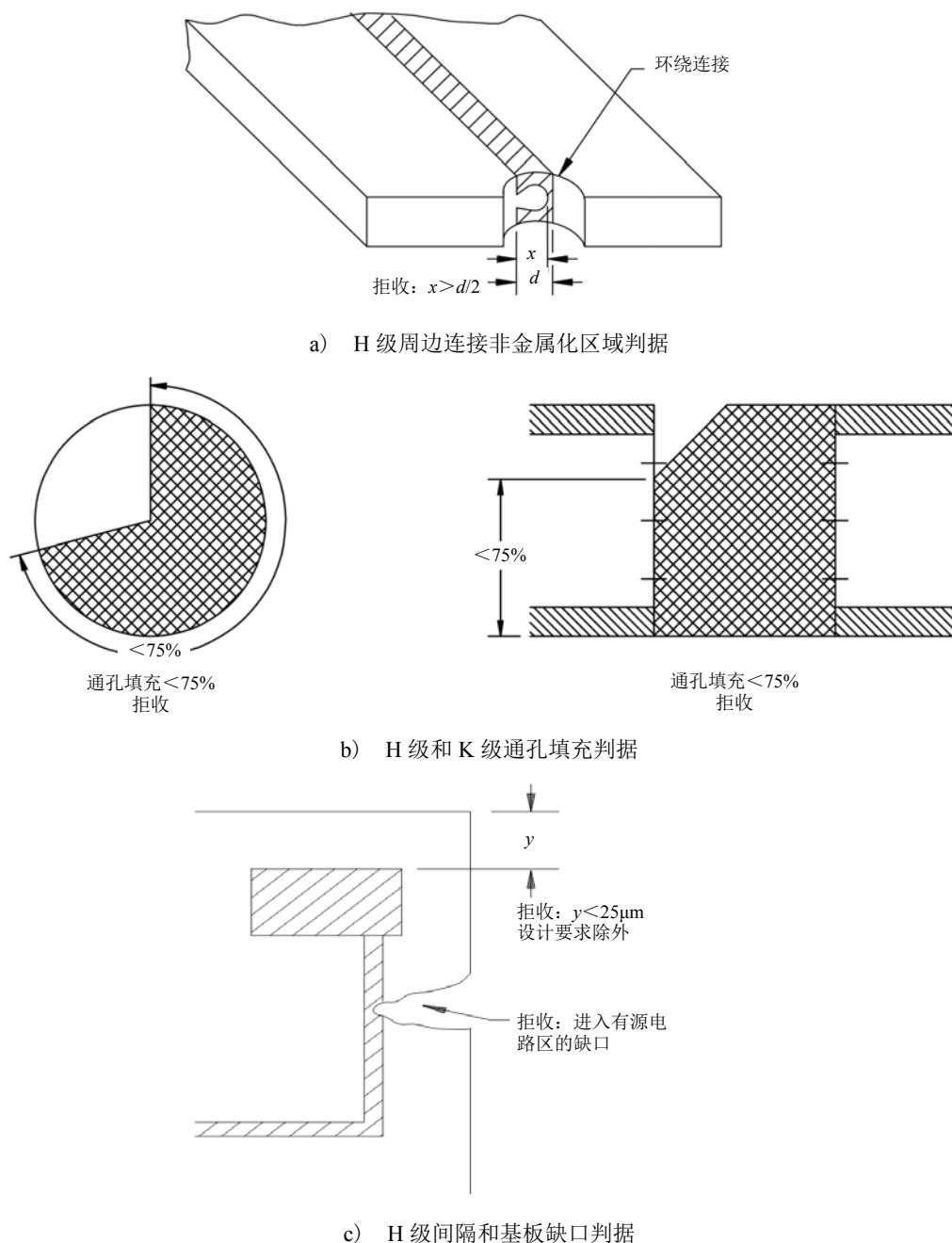
图 43 周边连接、基板通孔、基板缺陷判据
