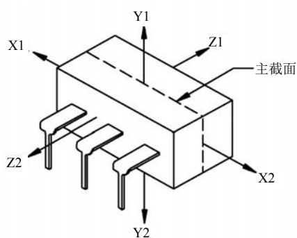
图3 双列封装
