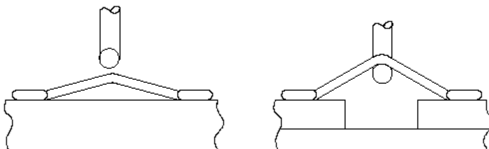
图 4 键合点在同一水平面的引线键合拉力试验
