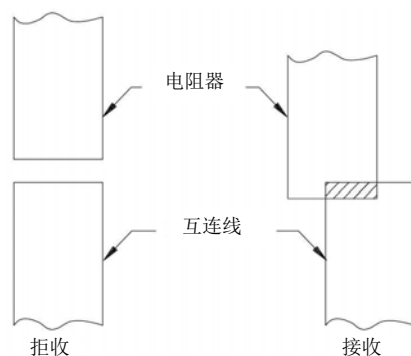
图 27 膜电阻器的接触区
