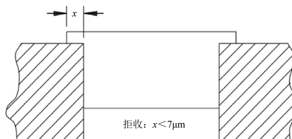
图 17 H 级接触重叠判据
