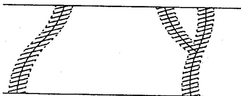
图 2 铝层上的玻璃钝化层中出现裂纹(B 类)
