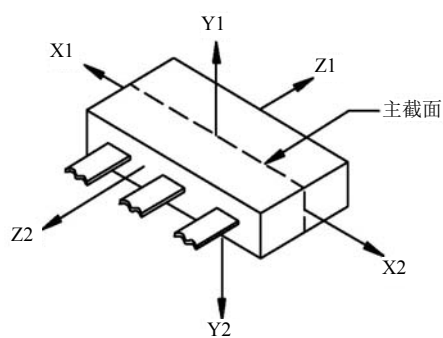
图4 单边径向引线的扁平封装
