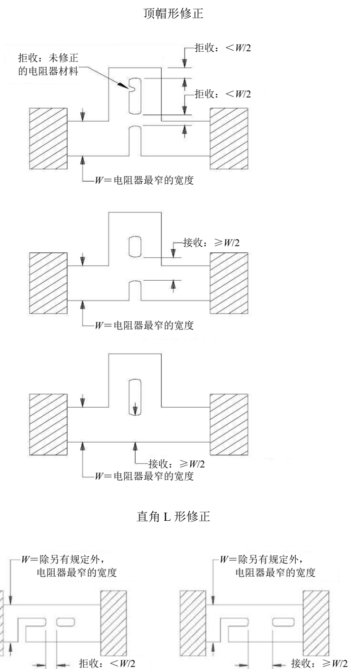
图 30 电阻器判据
