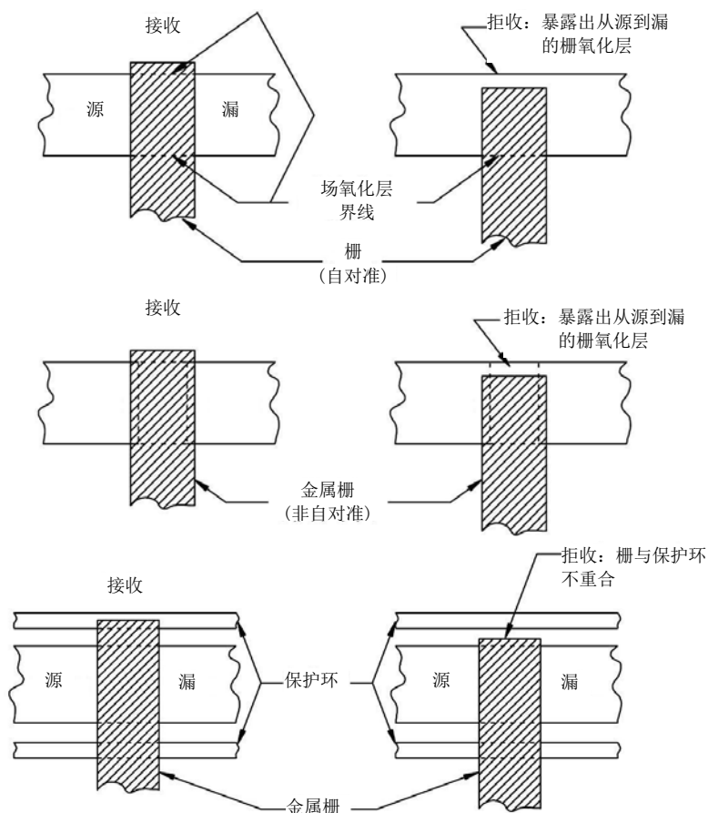
图 17 MOS 栅对准
