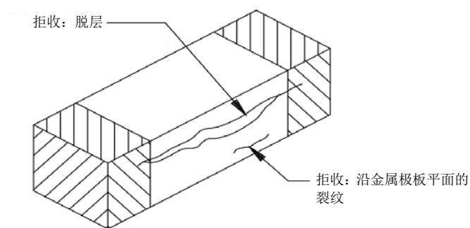
图 57 H 级脱层判据
