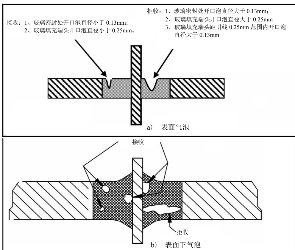
图 7 气泡
