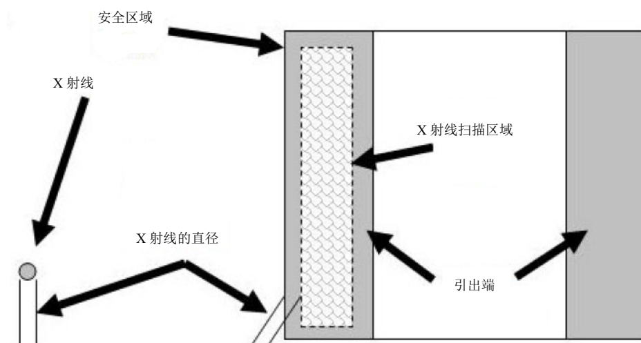
图1 较大平面扫描区域示例
