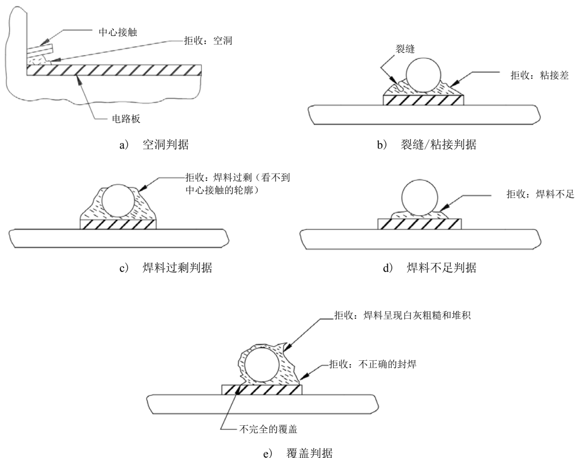
图 11 焊料判据
