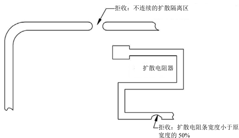
图 20 扩散缺陷
