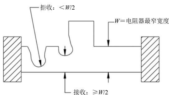
图 29 未修正的电阻器的划伤和空洞判据
