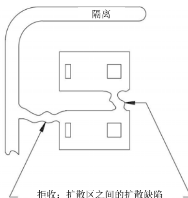
图 19 扩散缺陷
