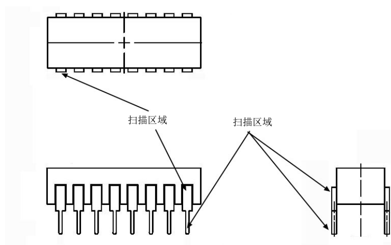
图 5 双列直插封装的扫描区域
