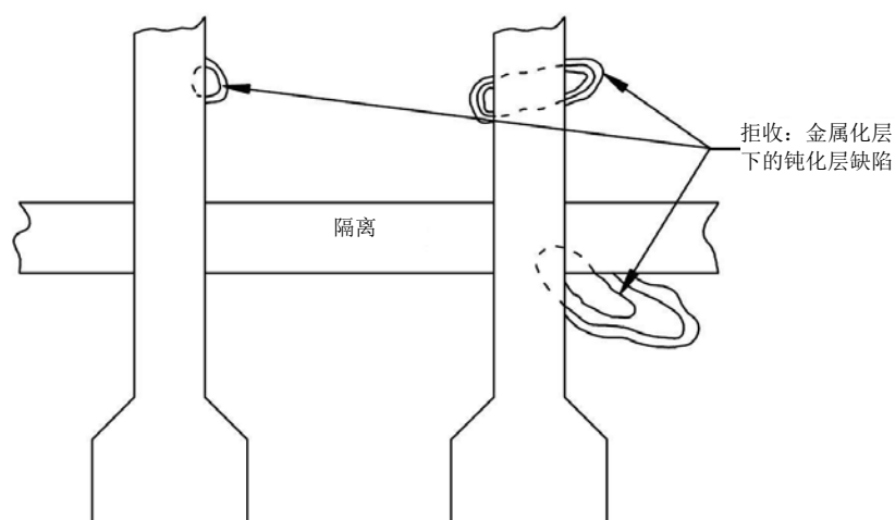
图 21 钝化层缺陷
