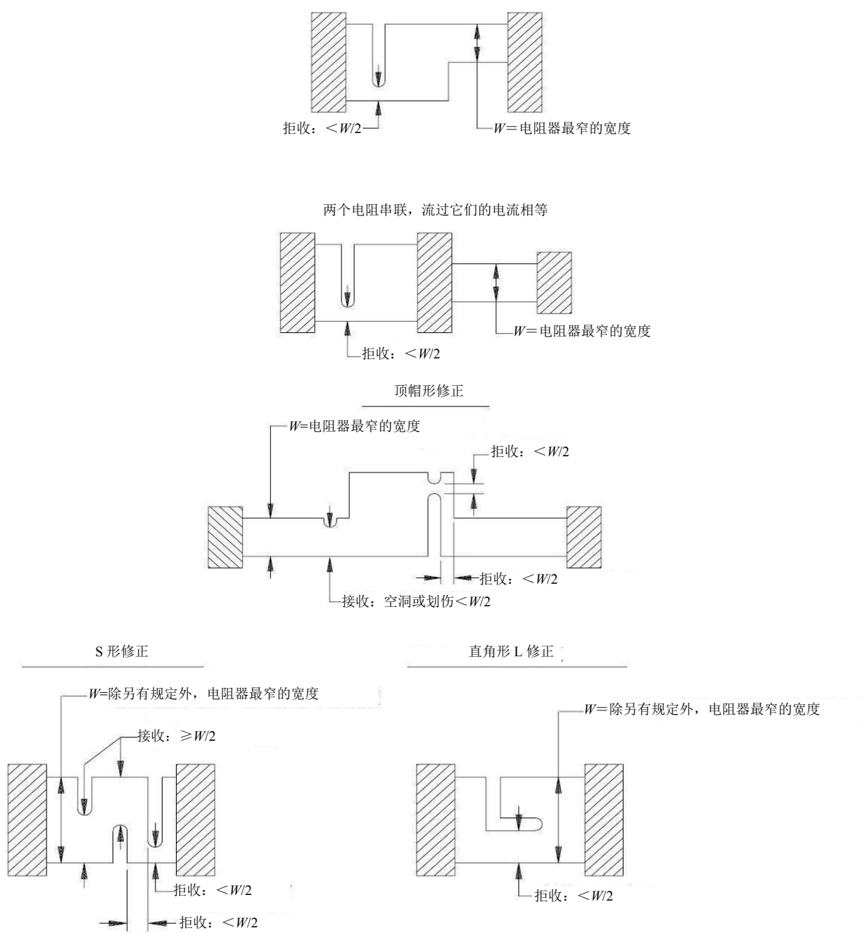
图 31 电阻器划伤、空洞和修正判据
