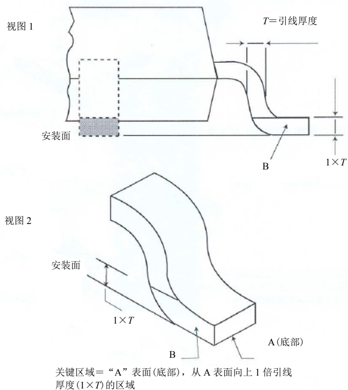
图 A.3 翼型引线器件
