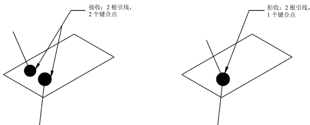
图 5 一个键合固定两根公用引线
