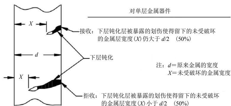
图5 B级的金属化层划伤判据
