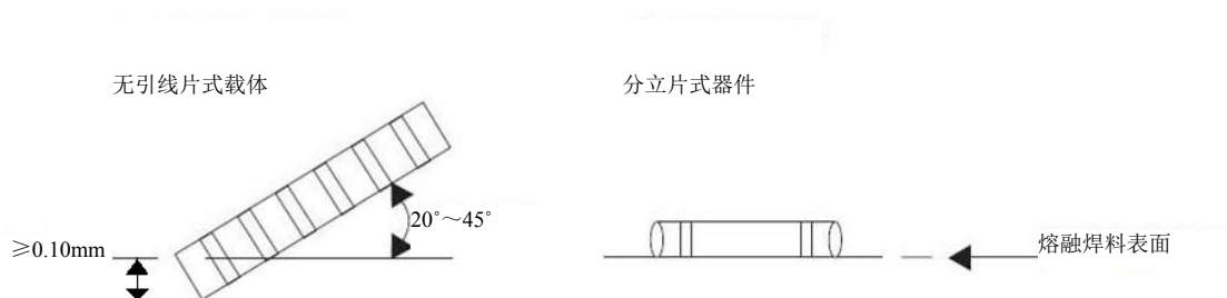
图4 无引线表面安装器件浸入深度
