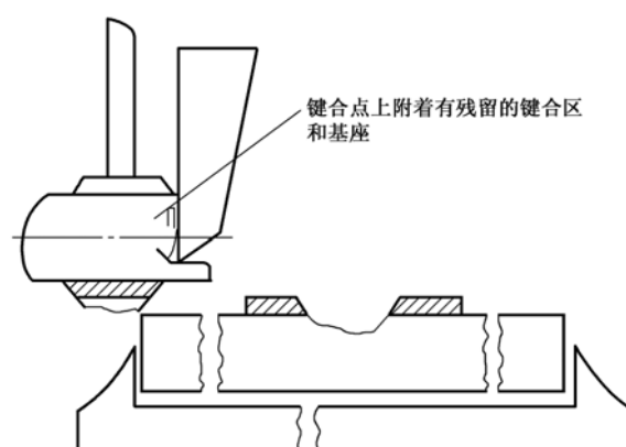
图 A. 4 凹坑
