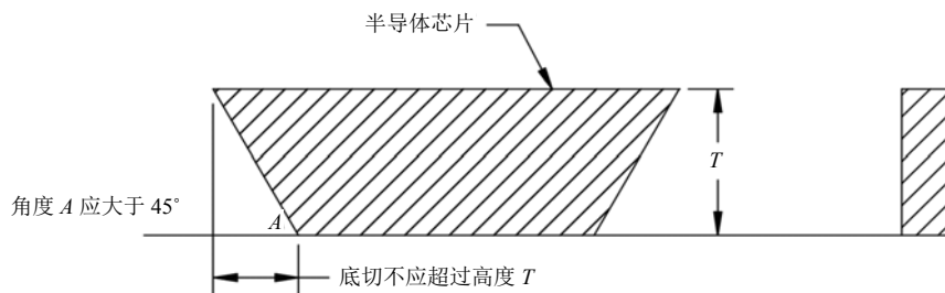
图5 底切
