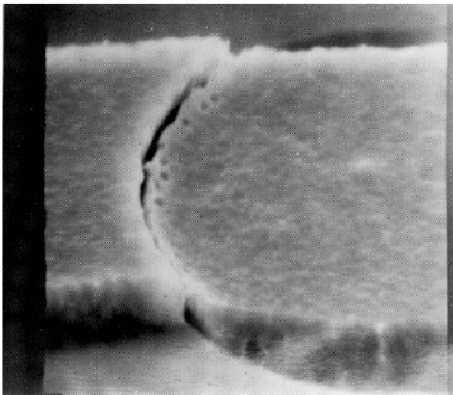
图 17 (9500 倍) 陡峭的钝化层台阶 (MOS) (拒收)
