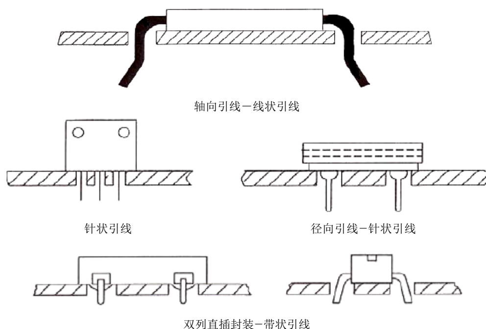
图 1 器件引线和安装示例
