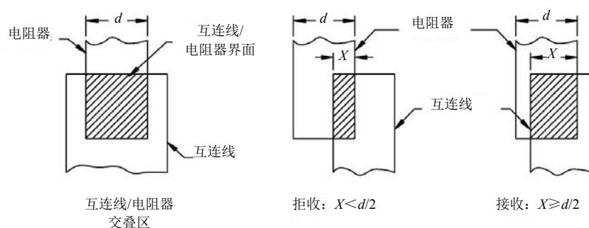
图 26 膜电阻器的接触区
