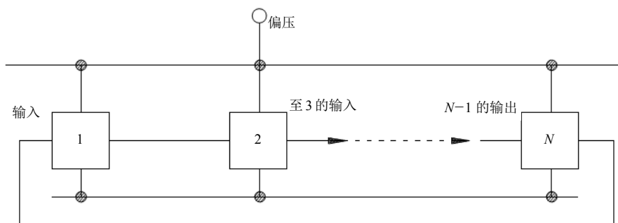
图 3 环形振荡器
