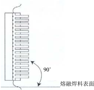
图 2 有引线表面安装器件浸焊料角度
