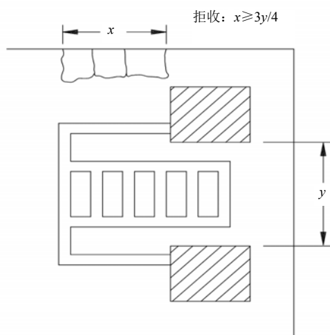
图 12 K 级半圆形裂纹判据
