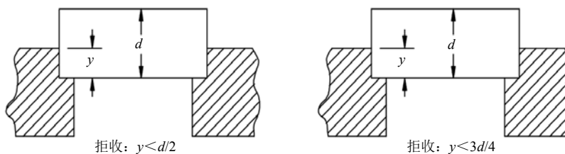
a) H 级电阻覆盖判据
