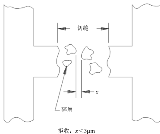
图 24 对于自钝化电阻材料碎屑的 H 级判据
