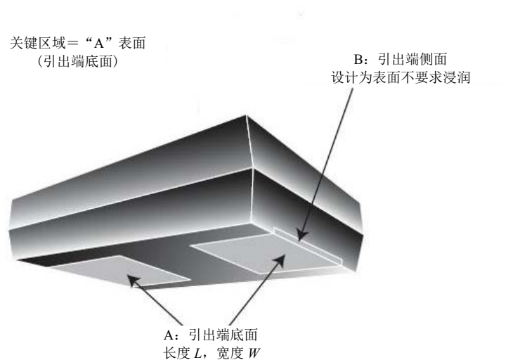
图 A.8 外露焊盘封装
