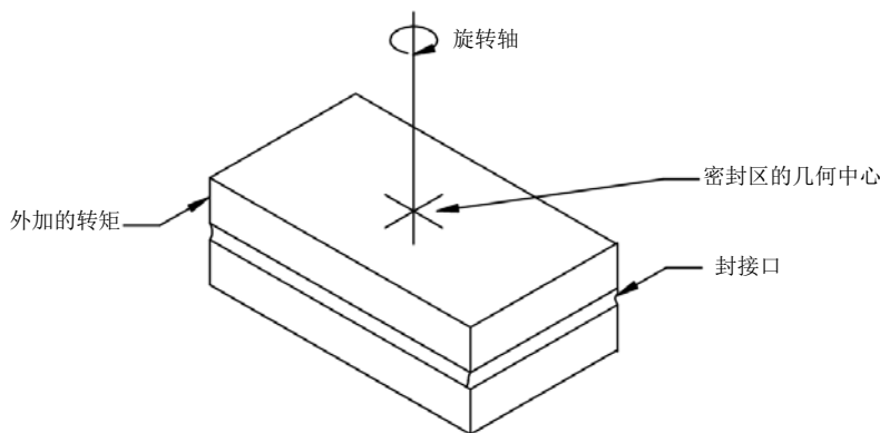
图1 扭矩的施加
