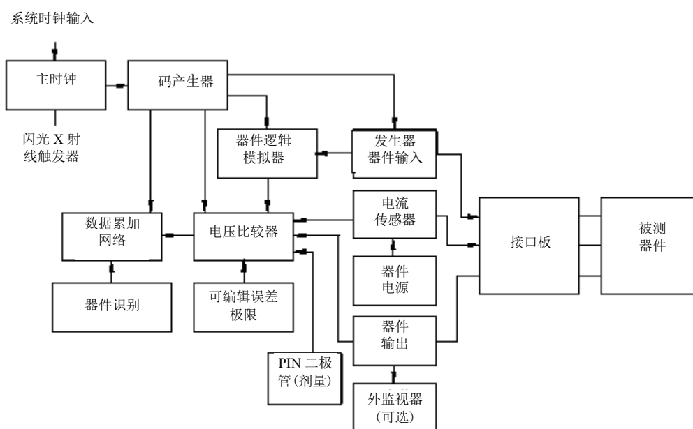
图1 锁定系统
