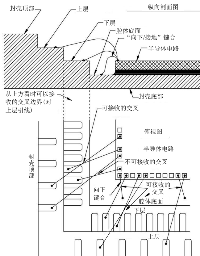
图 36 引线与引线交叉的 S 级判据
