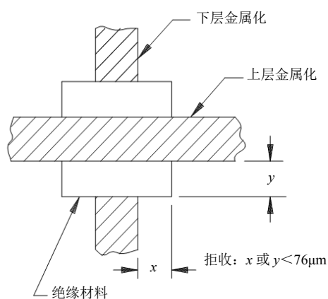
图 53 H 级绝缘材料扩展判据
