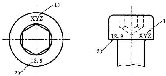
图 8 内六角圆柱头螺钉标志示例
