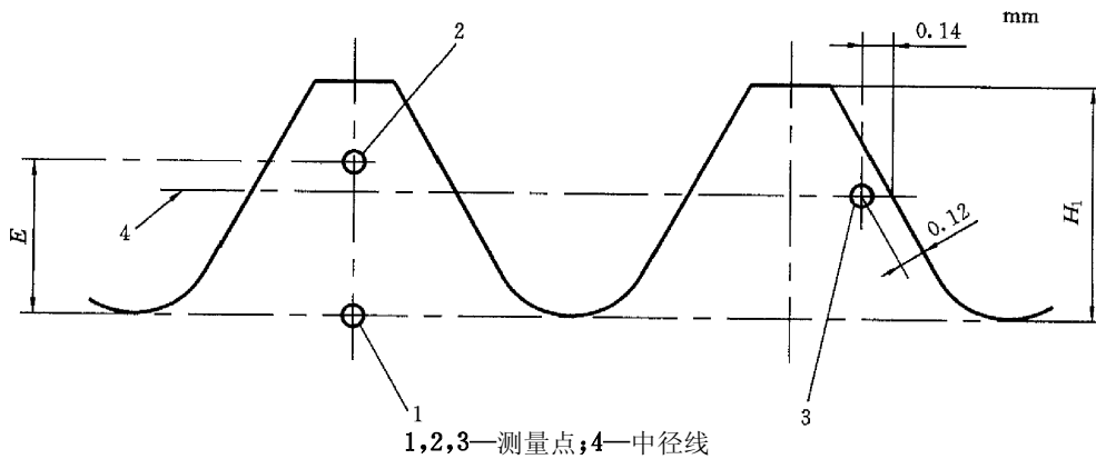
图 6 脱碳层试验的硬度测量法
