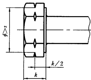
图 12 可选用的左旋螺纹的标志
