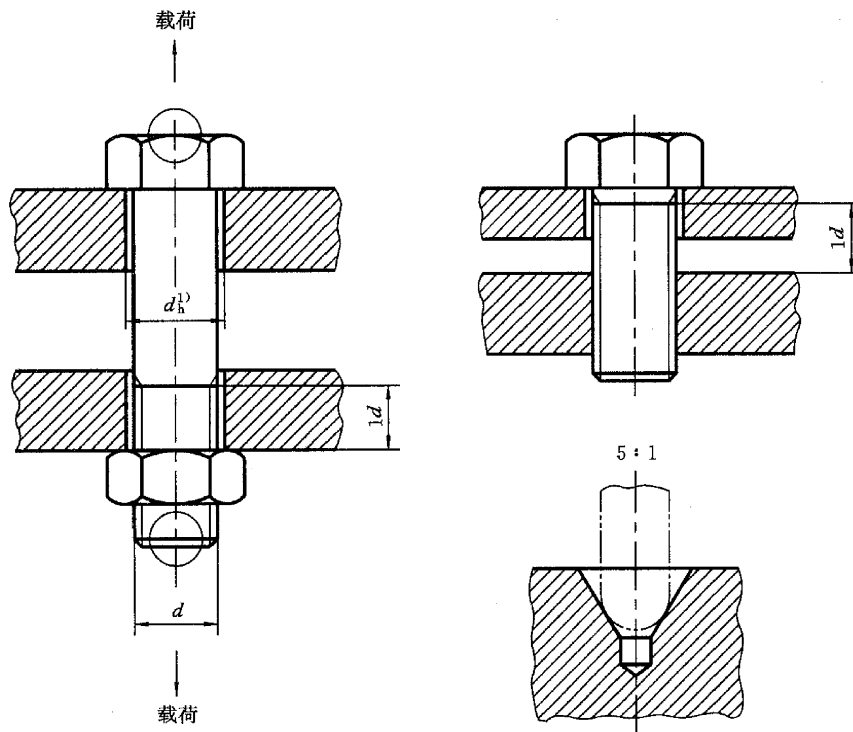
图 2 对紧固件实物施加保证载荷试验
