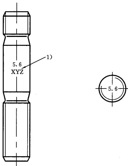
图 10 螺栓标志示例
