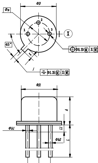
图 1 器件 (A3-02B 型) 外形图
